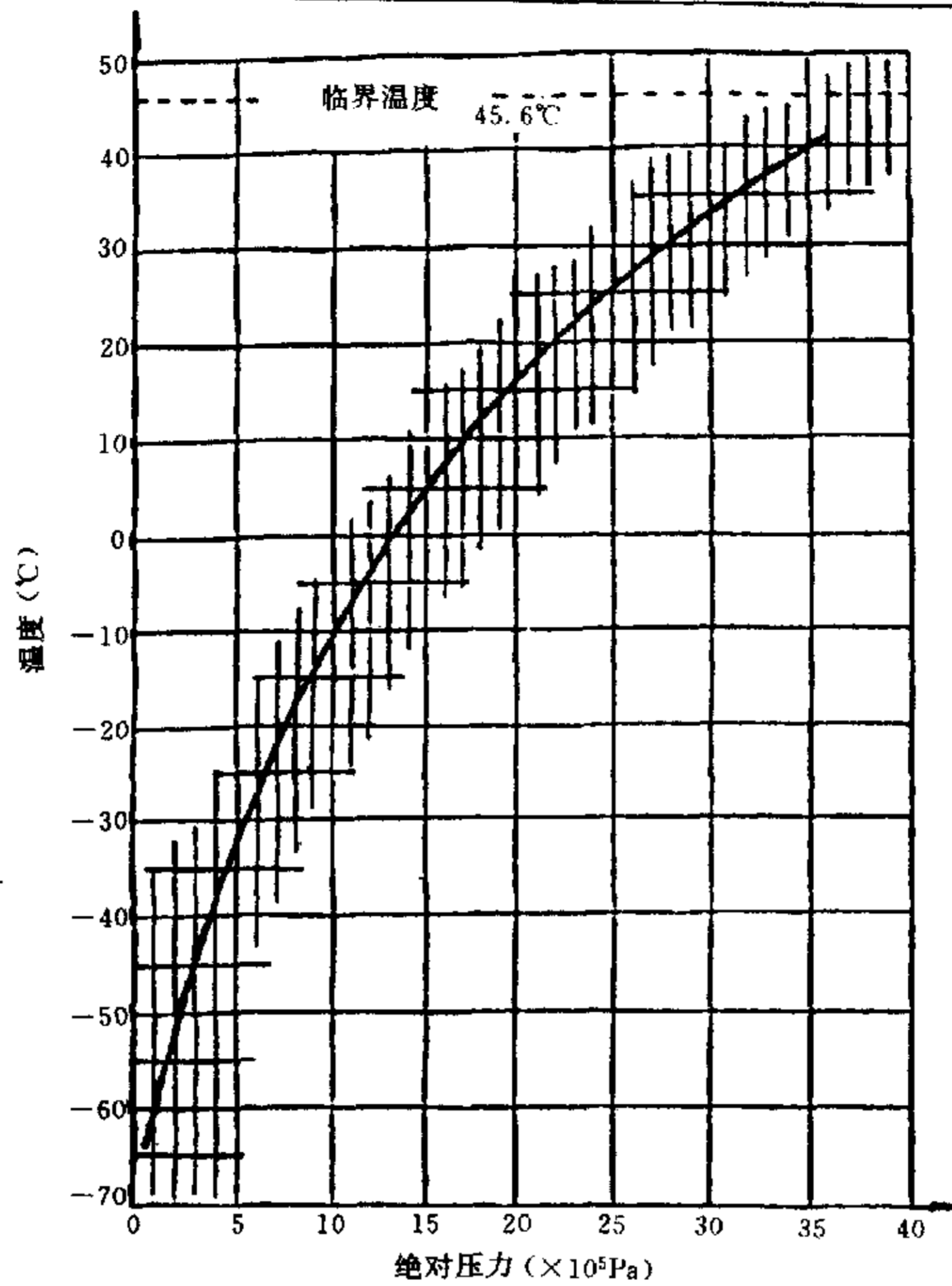
图 1 六氟化硫的饱和蒸汽压曲线
